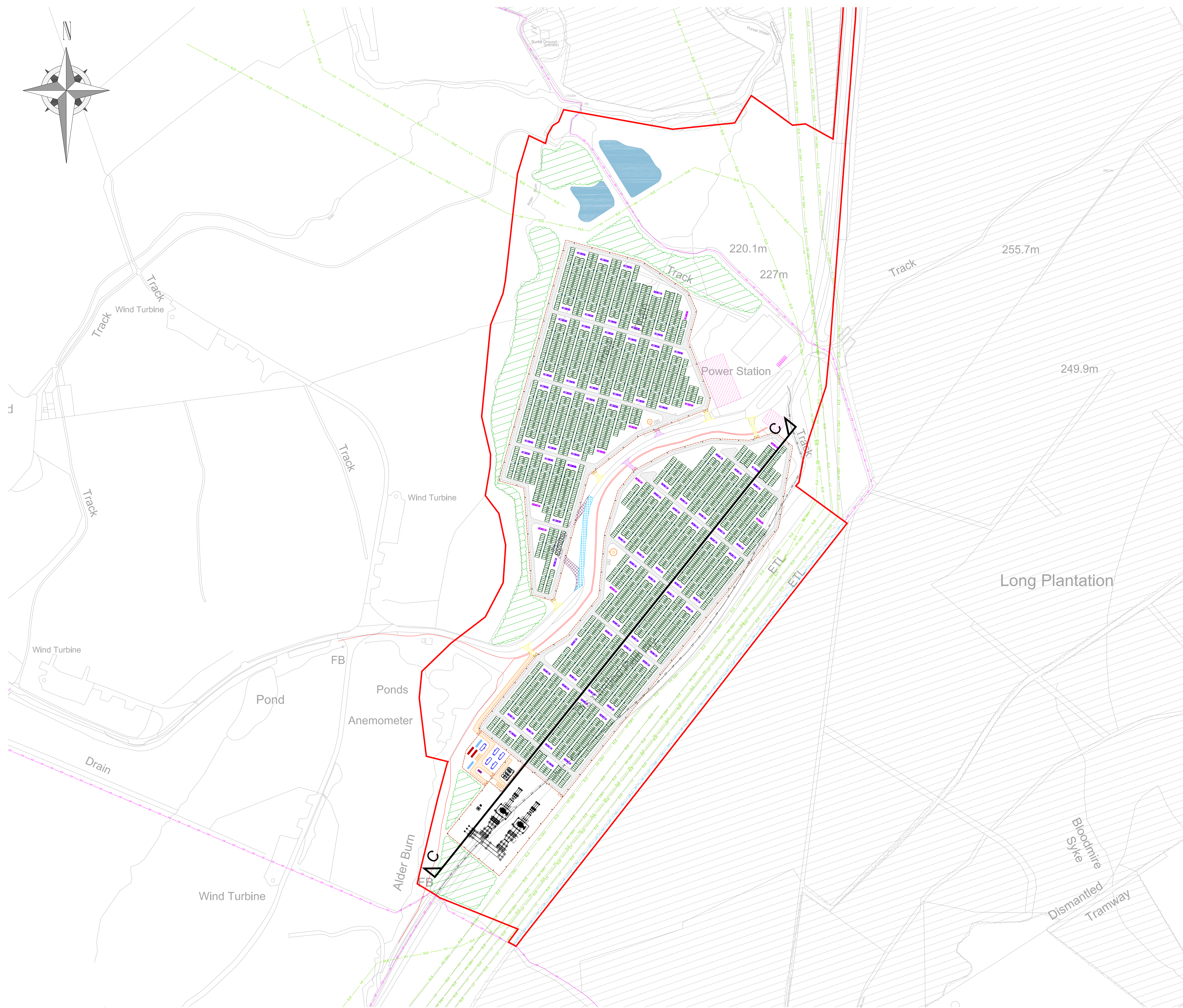
1 KEY PLAN Scale: 1:1250@A0
