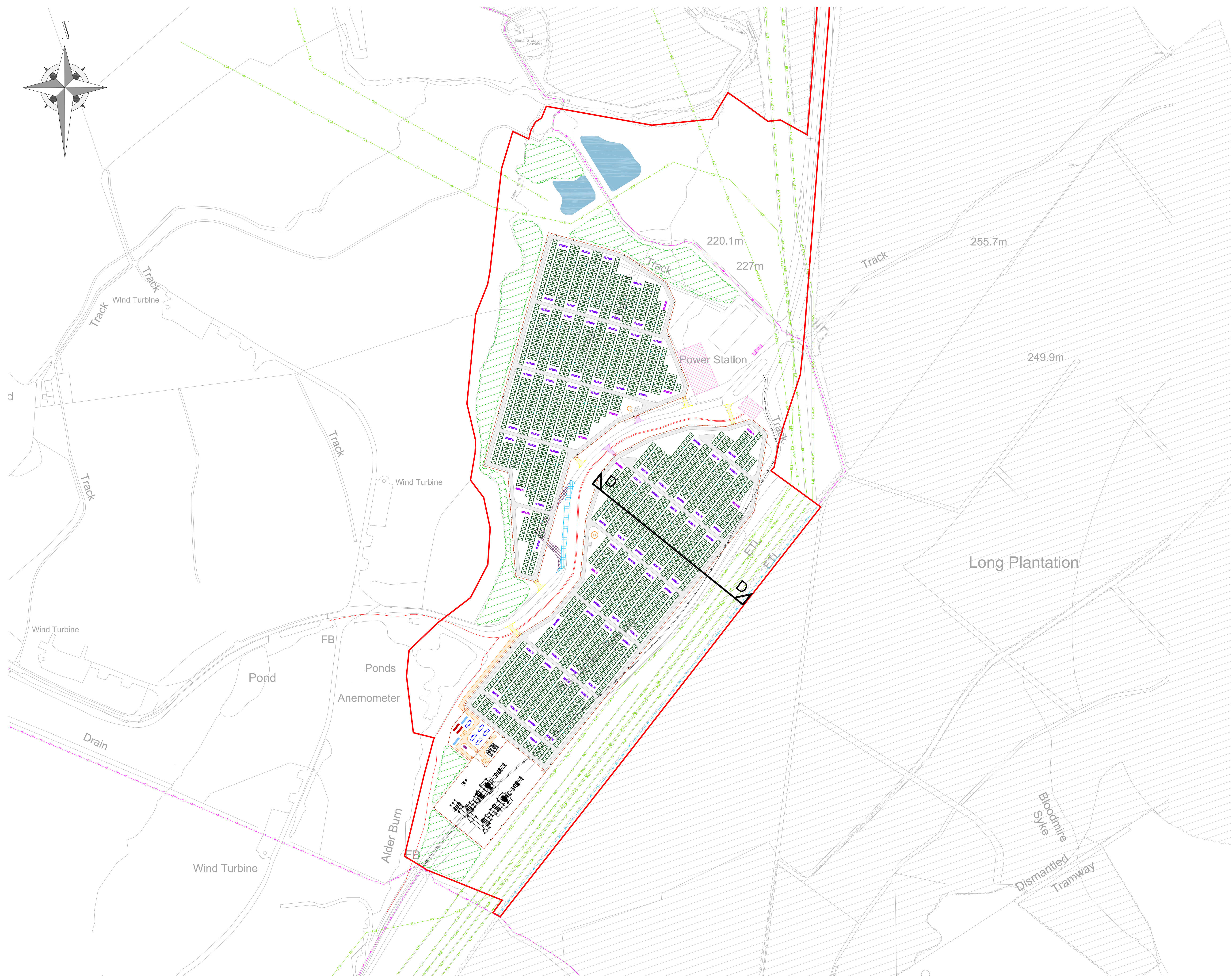
1 KEY PLAN Scale: 1:1250@A0
